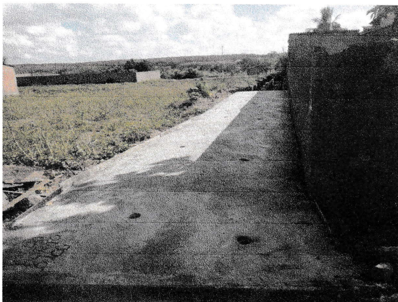
FIGURA 4 – EXECUÇÃO DE FORMAS E ARMAÇÃO DE LAJES E VIGAMENTOS DO TRECHO ENTRE A RUA BEVENUTO ALVES DA ROCHA E A RUA VICENTE DAS CHAGAS DE OLIVEIRA
