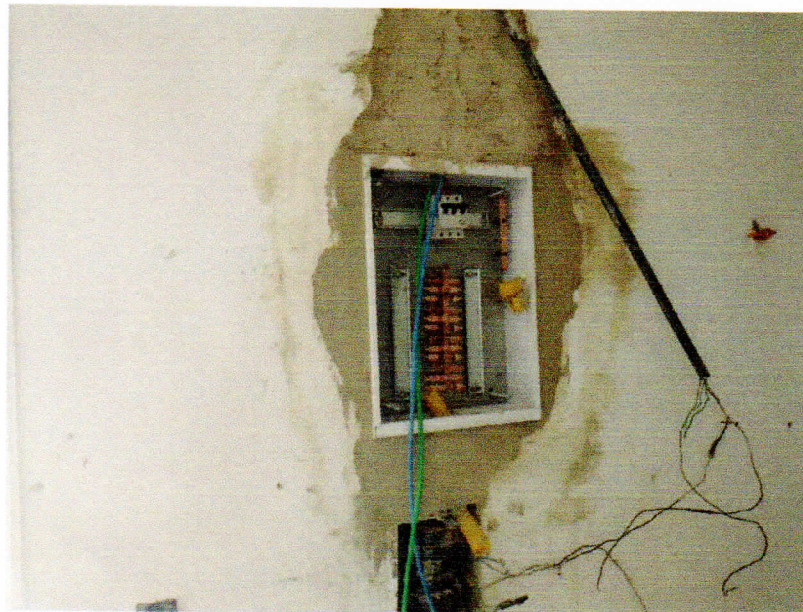
Figura 16 – EXECUÇÃO DE QUADRO DE DISTRIBUIÇÃO;
