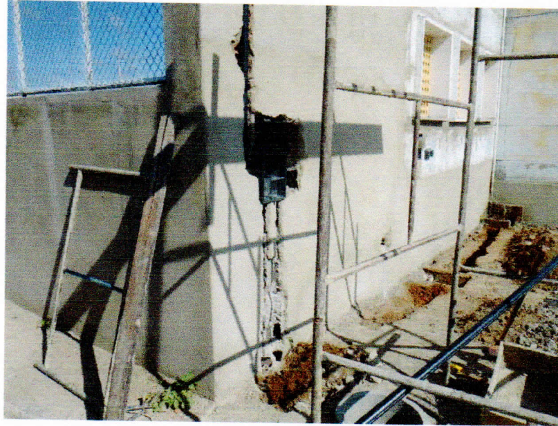
FIGURA 11 – EXECUÇÃO DE PADRÃO DE ENTRADA DE ENERGIA;
