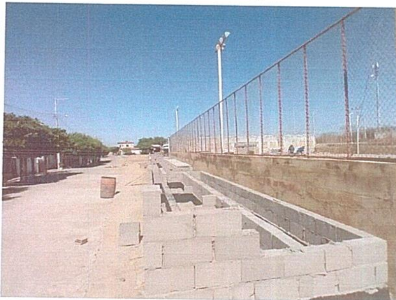
Figura 2 – EXECUÇÃO DE ALVENARIA EM BLOCOS DE CONCRETO (ARQUIBANCADAS);
