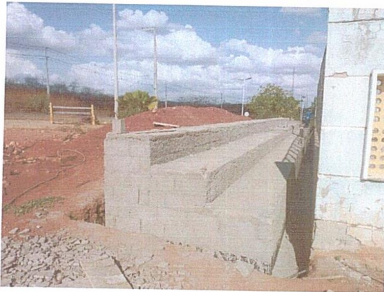
Figura 6 - EXECUÇÃO DE CHAPISCO E ASSENTAMENTO DE LAJES PRÉ-FABRICADAS;
