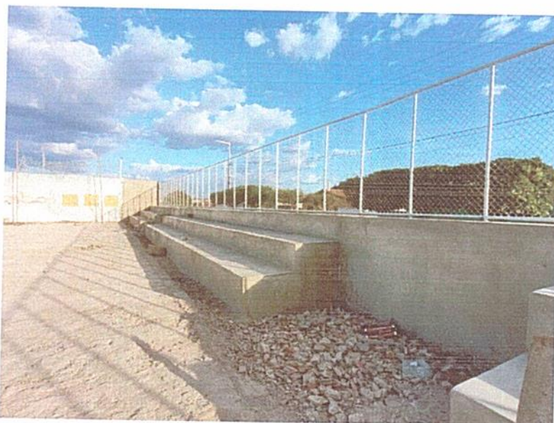
Figura 7 – EXECUÇÃO DE REBOCO EM ARQUIBANCADAS;
