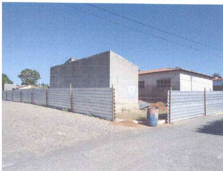
Figura 4 - TAPUMES COM TELHAS METALICAS;
