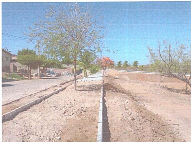
FIGURA 8 - EXECUÇÃO DE SERVIÇOS DE ASSENTAMENTO DE GUIA (MEIO-FIO) EM CONCRETO;
