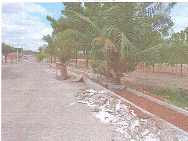
FIGURA 10 - EXECUÇÃO DE SERVIÇOS DE ASSENTAMENTO DE GUIA (MEIO-FIO) EM CONCRETO;
