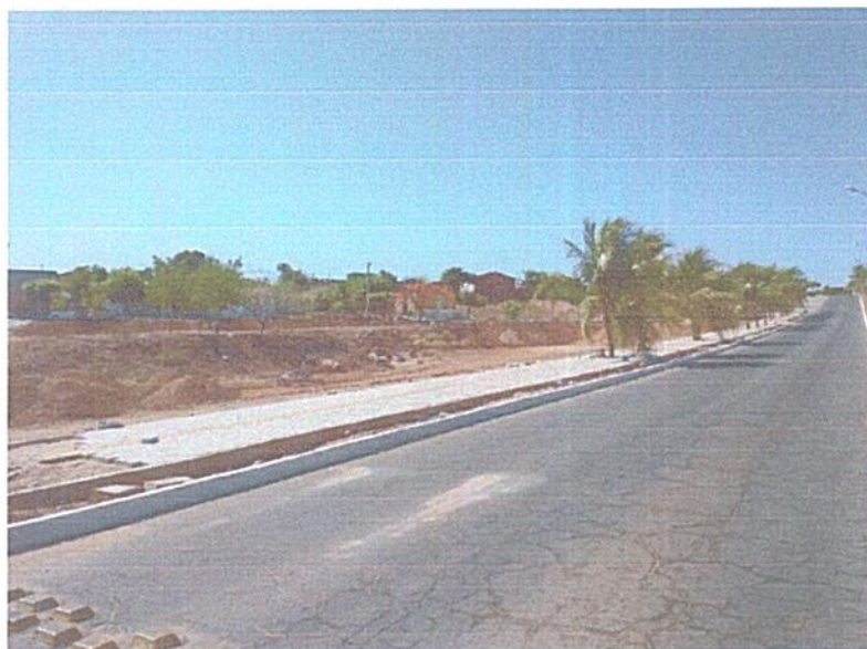
FIGURA 9 – EXECUÇÃO DE SERVIÇOS DE ASSENTAMENTO DE GUIA (MEIO-FIO) EM CONCRETO;
