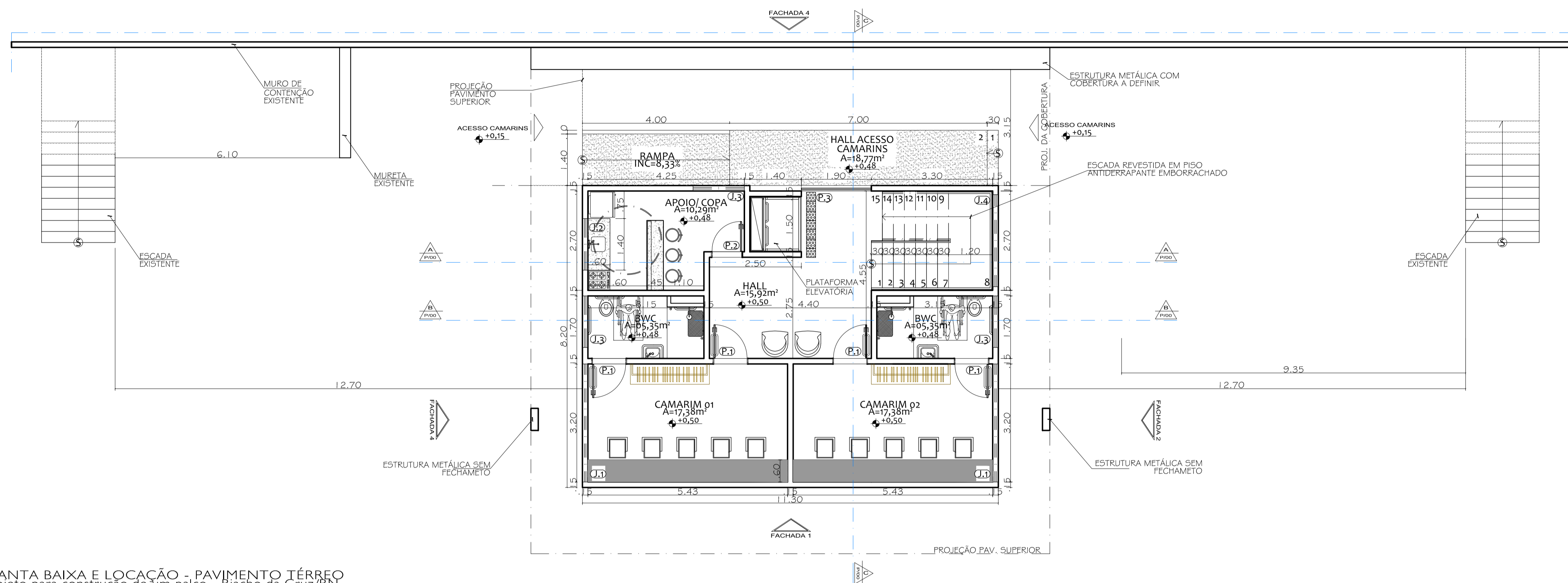
PLANTA BAIXA E LOCAÇÃO - PAVIMENTO TÉRREO Projeto para construção de um palco - Riacho da Cruz/RN Esc: 1/75
