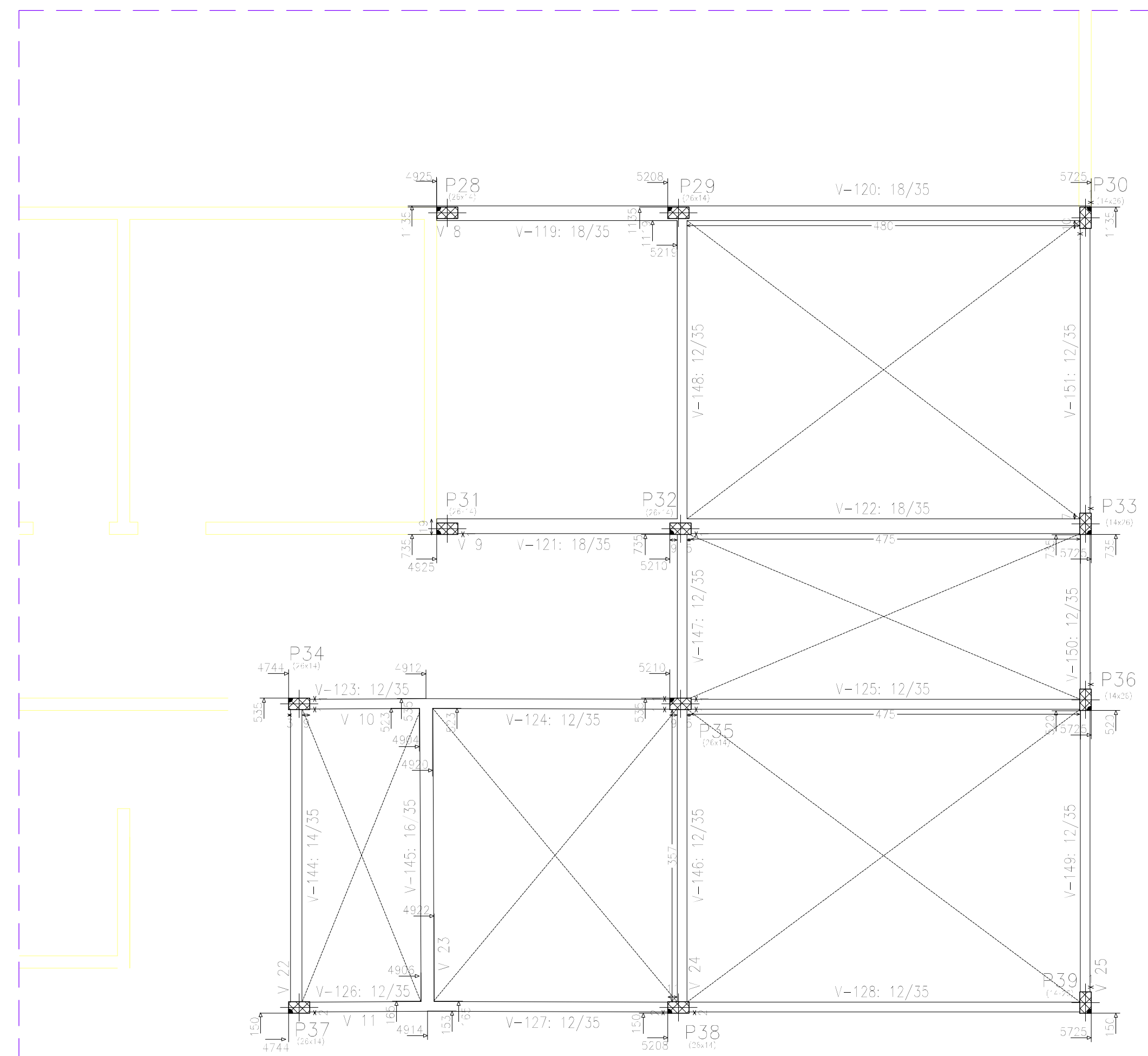
SETOR 2 Ampliação do Hospital Maternidade - Riacho da Cruz/RN Escala: 1/50
